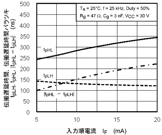
図 13.2.12 t_{pLH}, t_{pHL}, |t_{pHL} - t_{pLH}| - I_F
