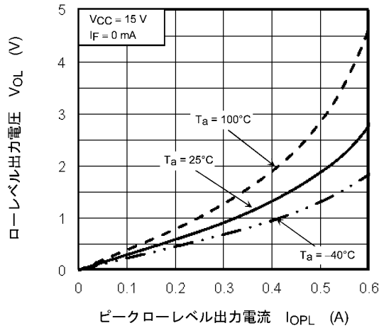
図 13.2.9 V_{OL} - I_{OPL}
