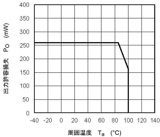
図 13.2.3 P_O - T_a
