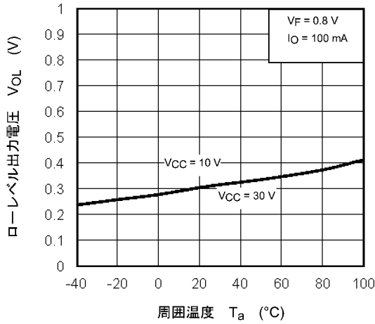
図 13.2.7 V_{OL} - T_a
