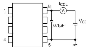
図 13.1.6 I CCL 測定回路
