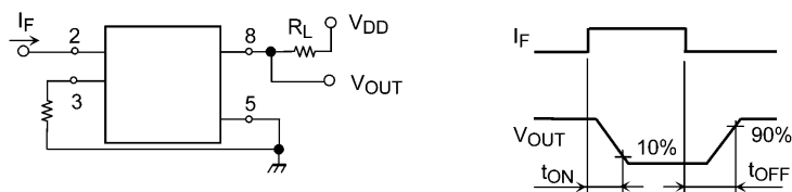
図 15.1 スイッチング時間測定回路, 波形
