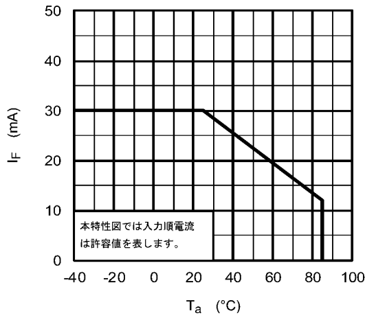
図 16.1.1 I_F - T_a
