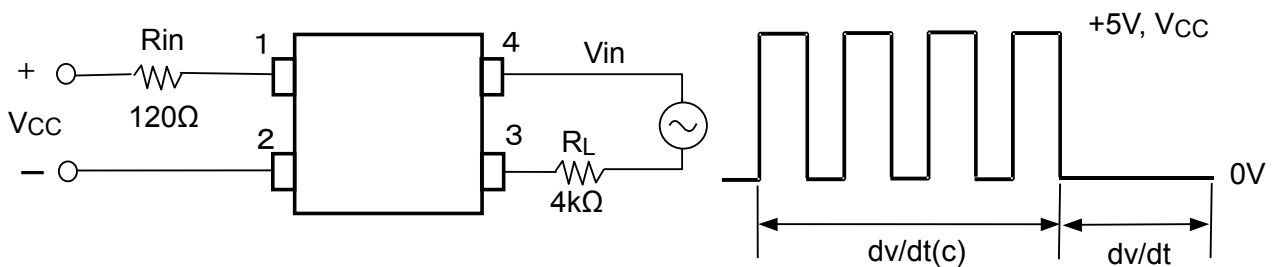
図 1: dv/dt 測定回路
