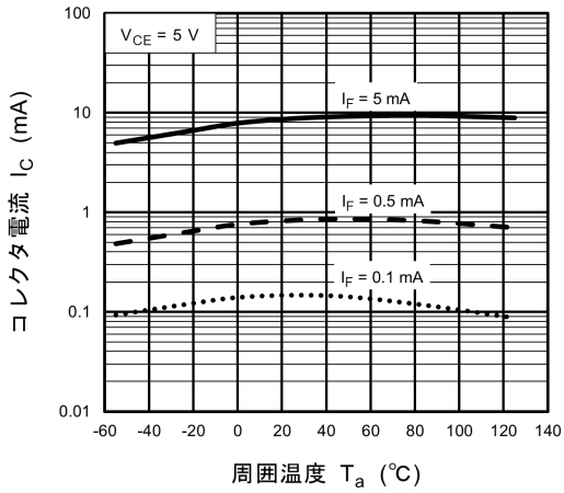
図 11.13 I_C - T_a
