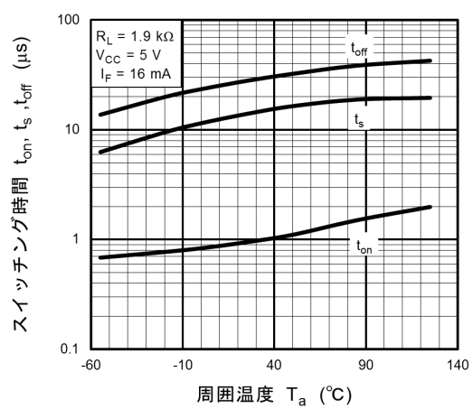
図 11.16 スイッチング時間 - T_a
