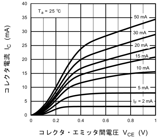
図 11.8 I_C - V_{CE}
