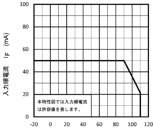
周囲温度 T_a (°C) 図 11.1 I_F - T_a
