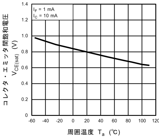
図 11.9 V_{CE(\text{sat})} - T_a
