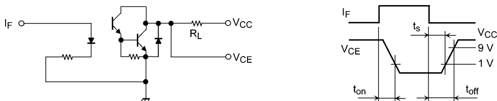
図 10.1 スイッチング時間測定回路, 波形
