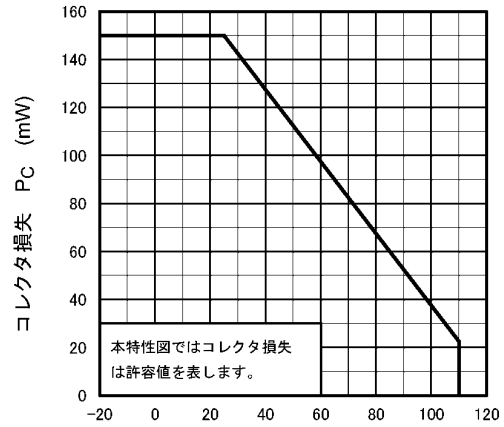
周囲温度 T_a (°C) 図 11.2 P_C - T_a
