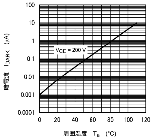
図 11.8 I_{\text{DARK}} - T_a
