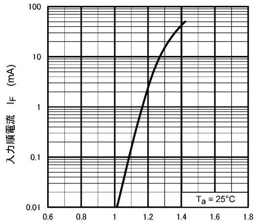
入力順電圧 V_F (V) 図 11.4 I_F - V_F
