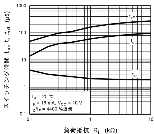
図 11.13 スイッチング時間 - R_L
