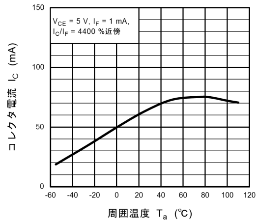
図 11.12 I_C - T_a
