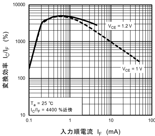
図 11.11 I_C/I_F - I_F
