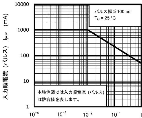
デューティ比 D_R 図 11.3 I_{FP} - D_R
