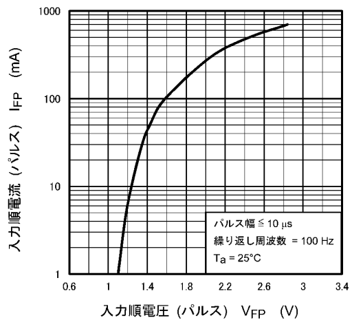
図 11.6 I_{FP} - V_{FP}
