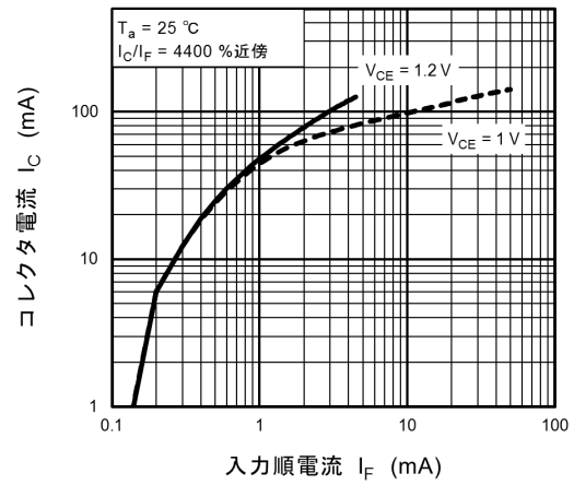
図 11.10 I_C - I_F
