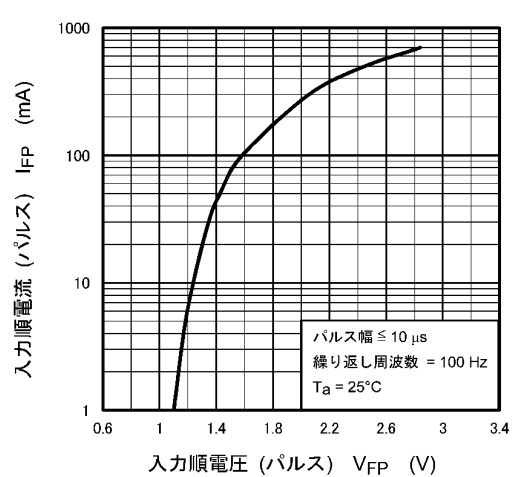
図 11.6 I_{FP} - V_{FP}
