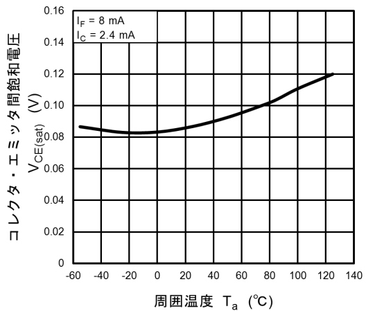
図 11.10 V_{CE(sat)} - T_a
