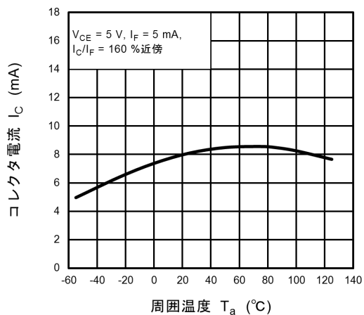
図 11.13 I_C - T_a
