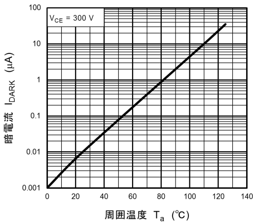
図 11.9 I_{DARK} - T_a
