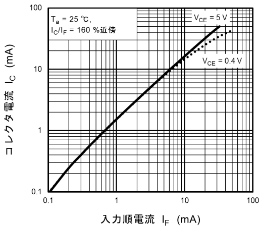
図 11.11 I_C - I_F
