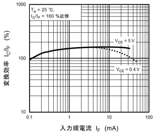
図 11.12 I_C/I_F - I_F
