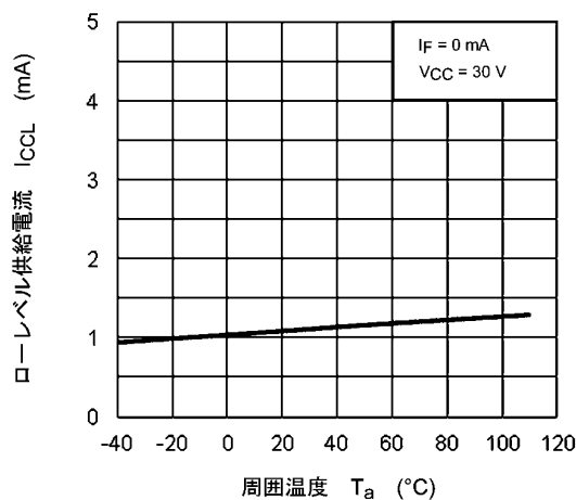
図 13.2.5 I_{CCL} - T_a
