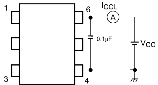
图 13.1.6 I CCL 测定回路
