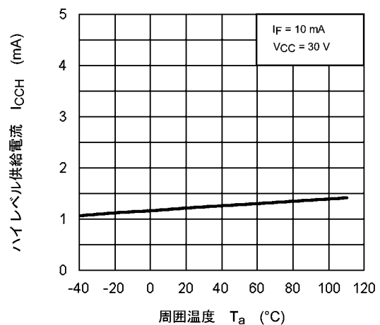
図 13.2.6 I_{CCH} - T_a
