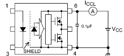
図 13.1.6 I CCL 測定回路
