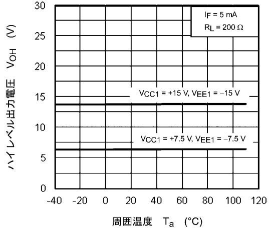
図 13.2.8 V_{OH} - T_a
