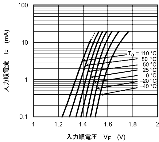
図 13.2.1 I_F - V_F
