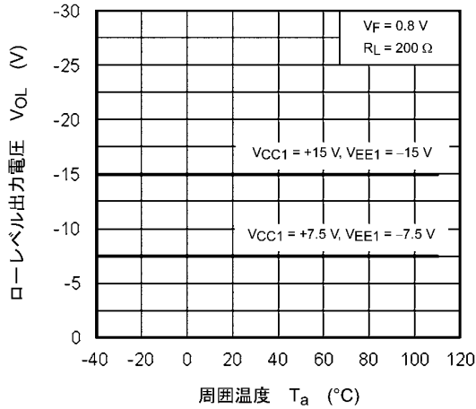
図 13.2.7 V_{OL} - T_a
