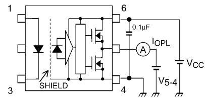
図 13.1.2 I OPL 測定回路
