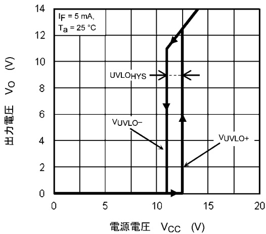
図 13.2.11 V_o(V_{UVLO}) - V_{CC}
