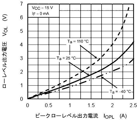
図 13.2.9 V_{OL} - I_{OPL}
