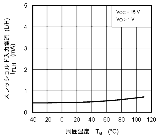
図 13.2.4 I_{FLH} - T_a
