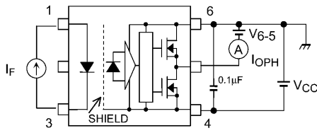
図 13.1.1 I OPH 測定回路
