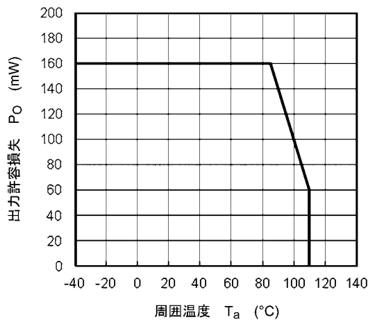
図 13.2.3 P_O - T_a
