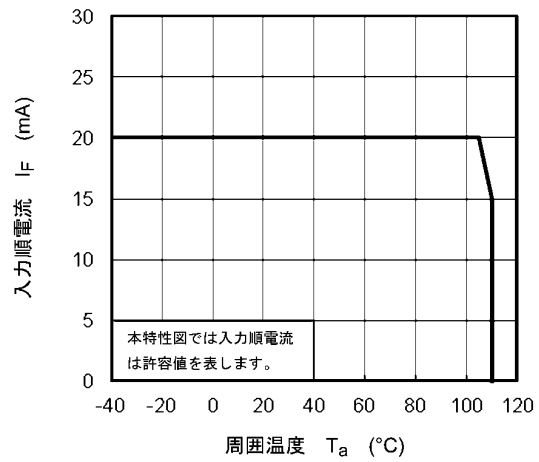
図 13.2.2 I_F - T_a
