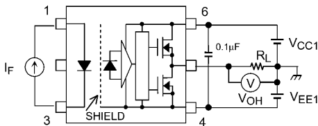
図 13.1.3 V OH 測定回路
