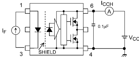
図 13.1.5 I CCH 測定回路
