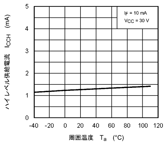
図 13.2.6 I_{CCH} - T_a
