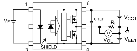
図 13.1.4 V OL 測定回路
