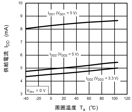
図 12.7 I_{DD} - T_a
