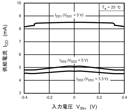
図 12.6 I_{DD} - V_{IN+}
