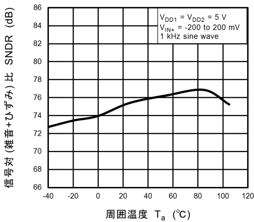
図 12.5 SNDR - T_a
