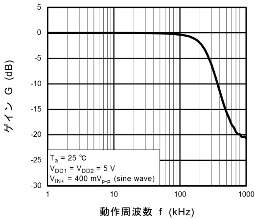
図 12.11 G[\text{dB}] - f
