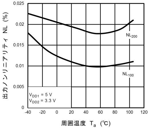
図 12.7 NL - T_a
