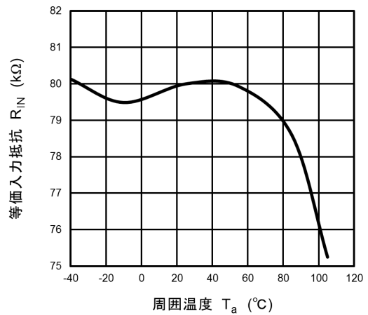
図 12.10 R_{IN} - T_a
