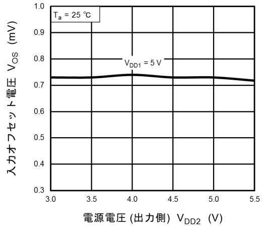
図 12.2 V_{OS} - V_{DD2}
