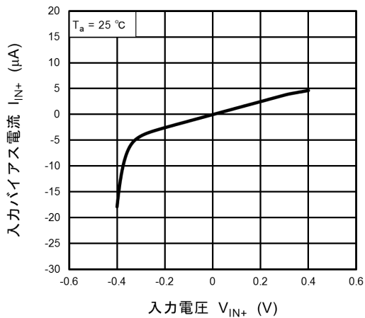
図 12.9 I_{IN+} - V_{IN+}
