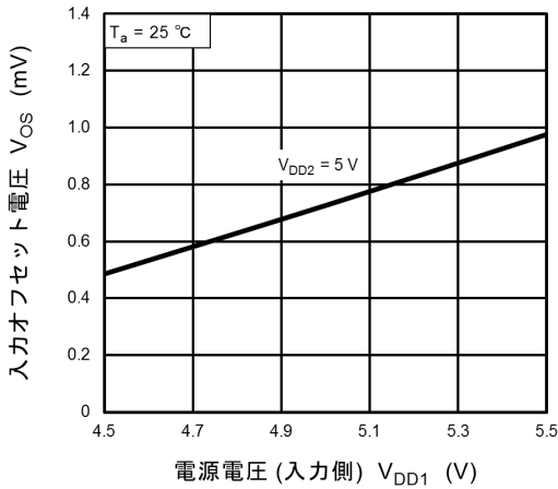
図 12.1 V_{OS} - V_{DD1}
