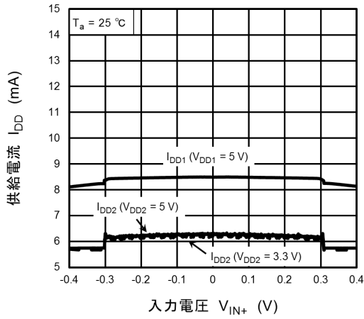
図 12.13 I_{DD} - V_{IN+}
