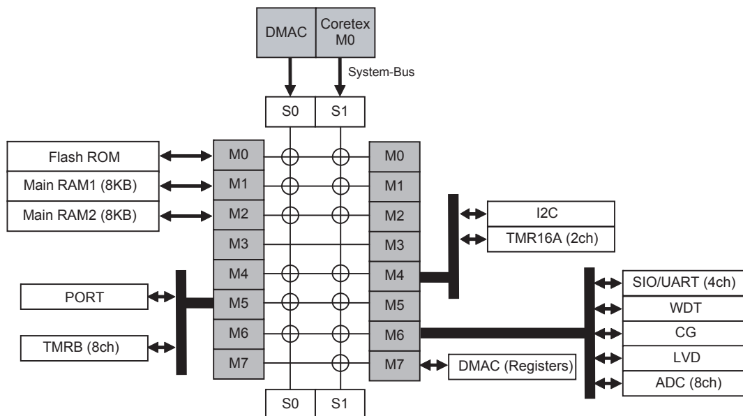
図 4-2 TMPM037FWUG (シングルチップモード)
