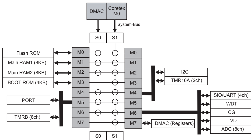
図 4-3 TMPM037FWUG (シングルブートモード)
