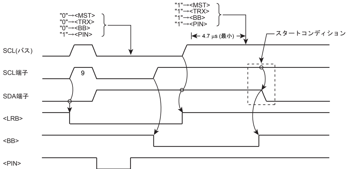
図 13-15 再スタートが発生する場合のタイミングチャート
