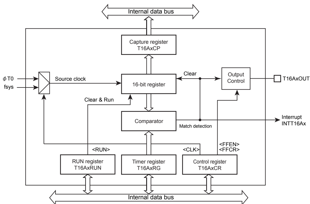
図 11-1 TMR16Ax ブロック図
