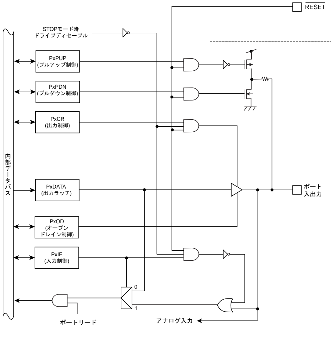
図 8-5 ポートタイプ FT5
