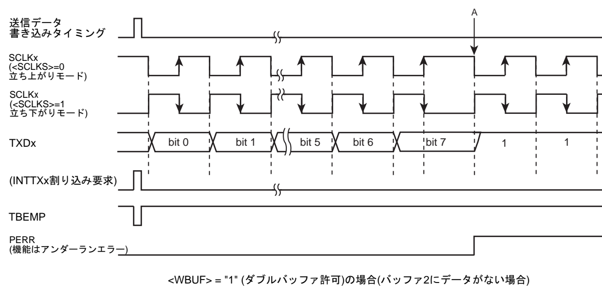
図 11-14 I/O インタフェースモード送信動作(クロック入力モード)
