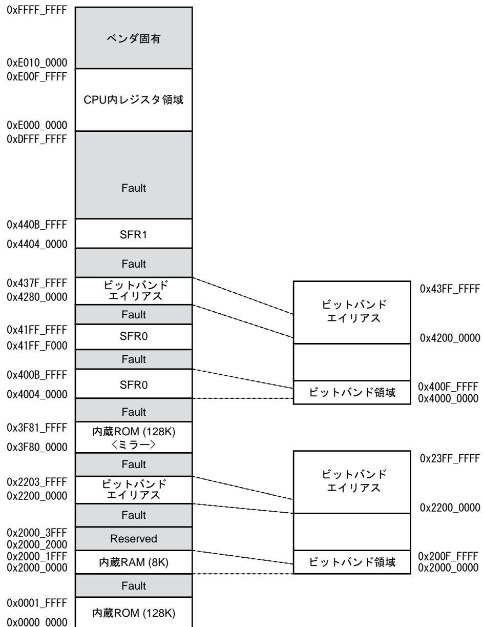
図 4-1 メモリマップ
