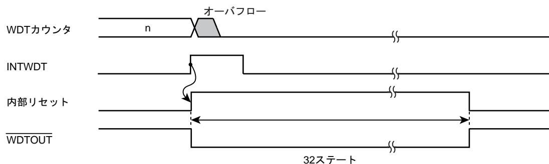
図 19-3 内部リセット発生
