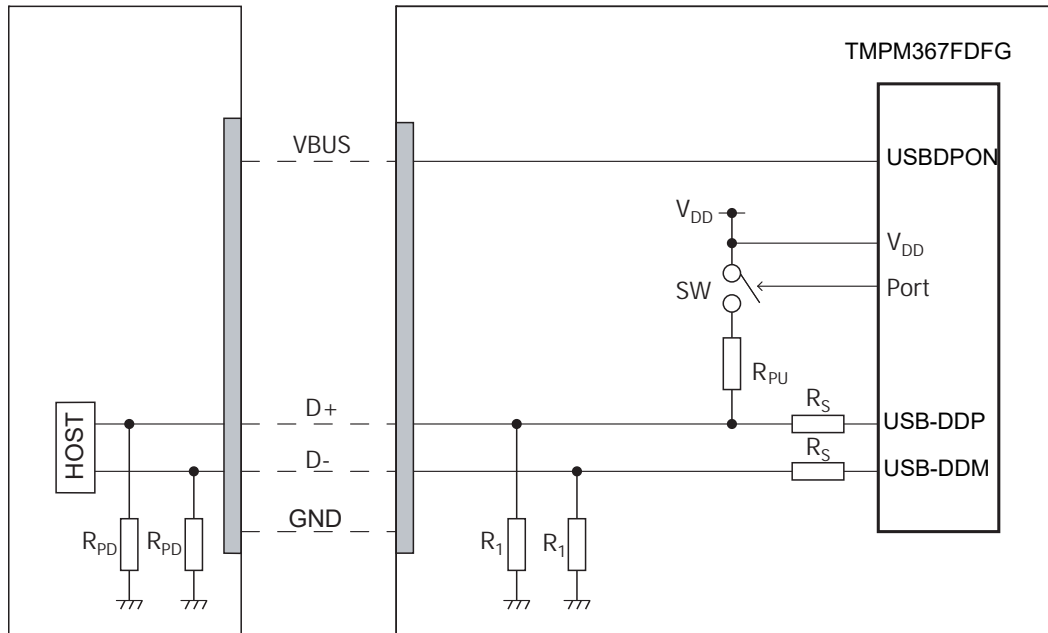
図 17-6 USB バスと TMPM367FDFG の接続例
