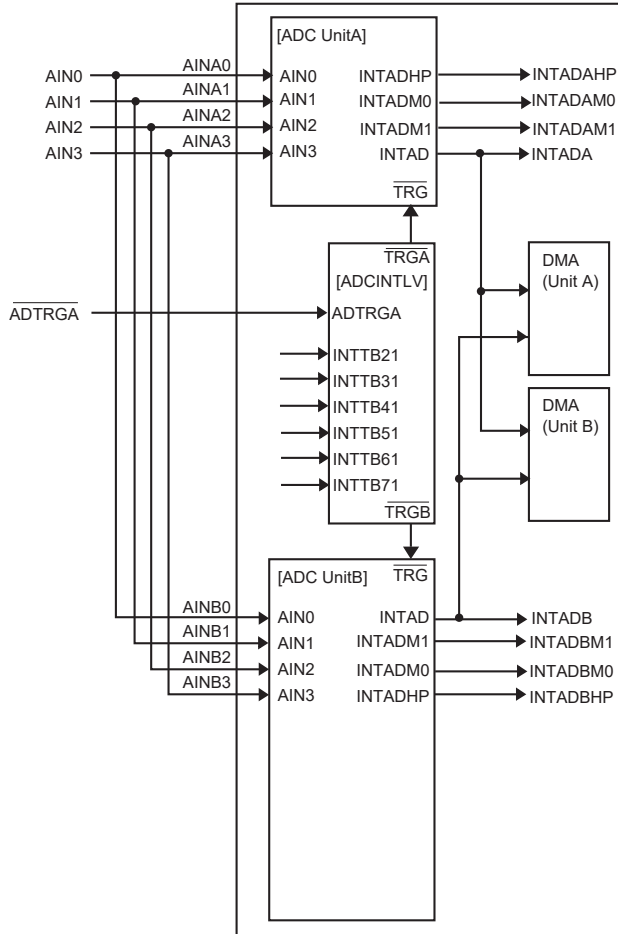
図 19-1 ブロック図 1
