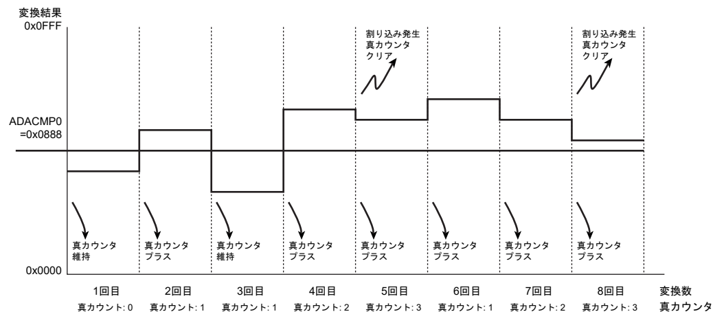
図 19-6 AD 監視機能（チャンネル固定リピート、判定カウント累積方式）
