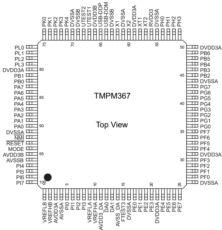
図 1-2 ピン配置図
