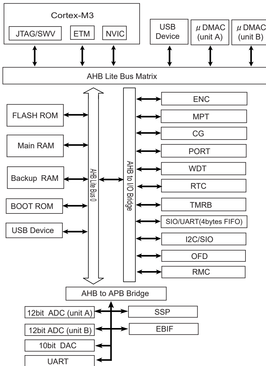
図 1-1 TMPM367FDFG ブロック図
