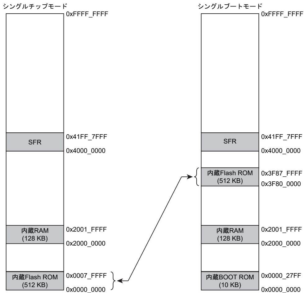
図 28-3 メモリマップの比較(TMPM367FDFG)
