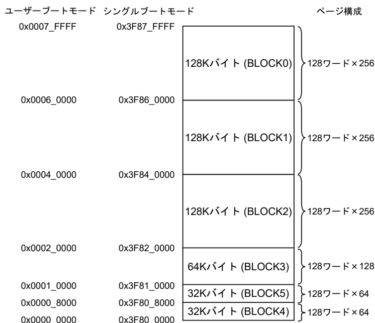
図 28-10 ブロック構成(TMPM367FDFG)
