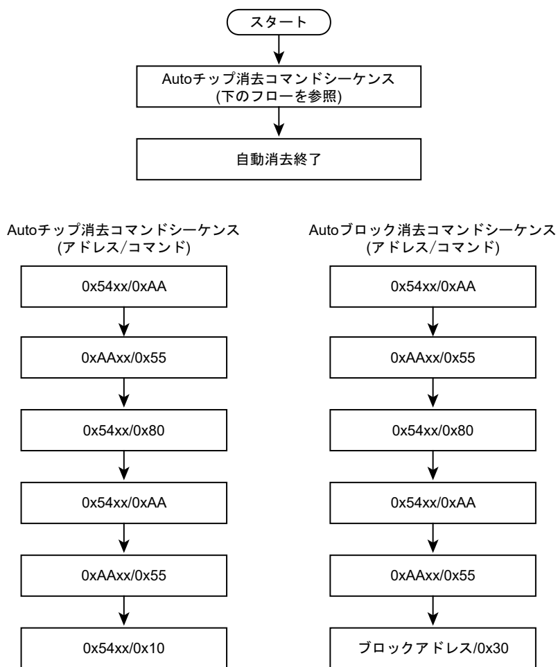
図 28-12 自動消去
