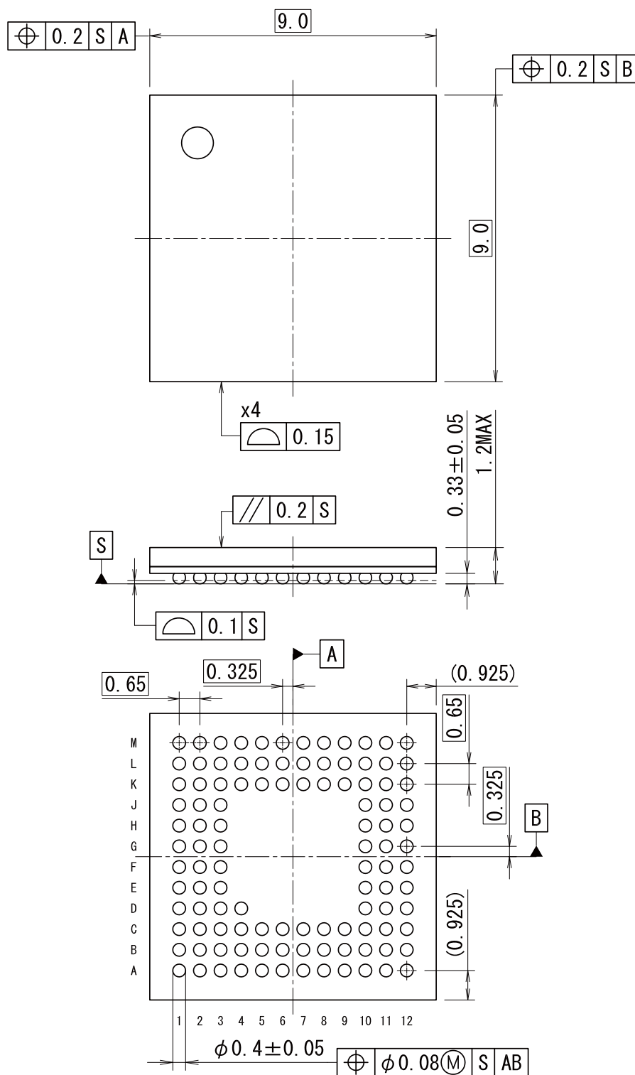
外形寸法図
