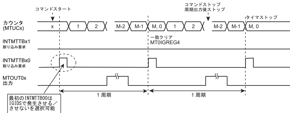
図 23-7 周期割り込み動作
