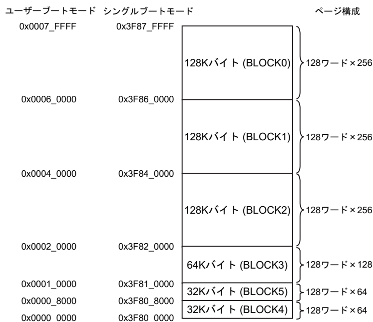
図 30-10 ブロック構成(TMPM368FDXBG)
