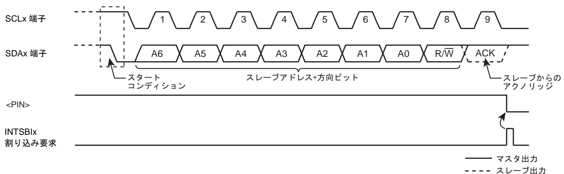
図 12-9 スタートコンディションとスレーブアドレスの発生
