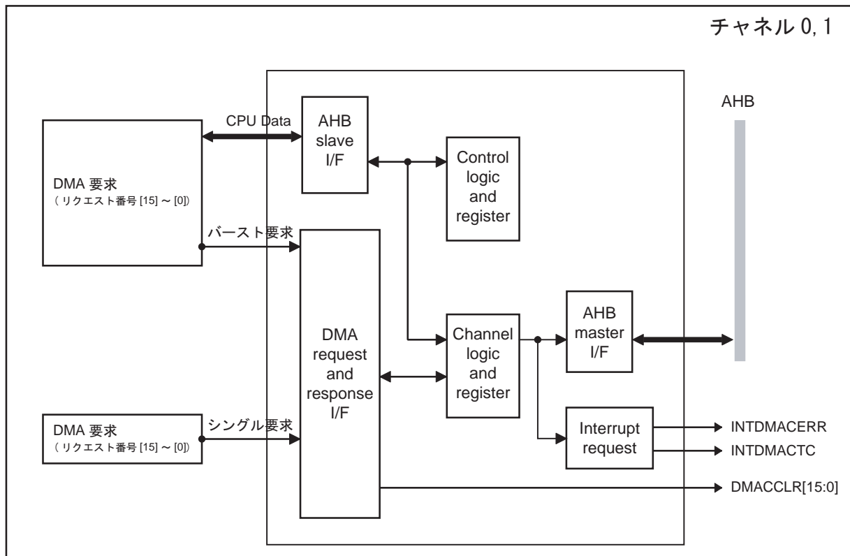
図 7-1 DMAC ブロック図
