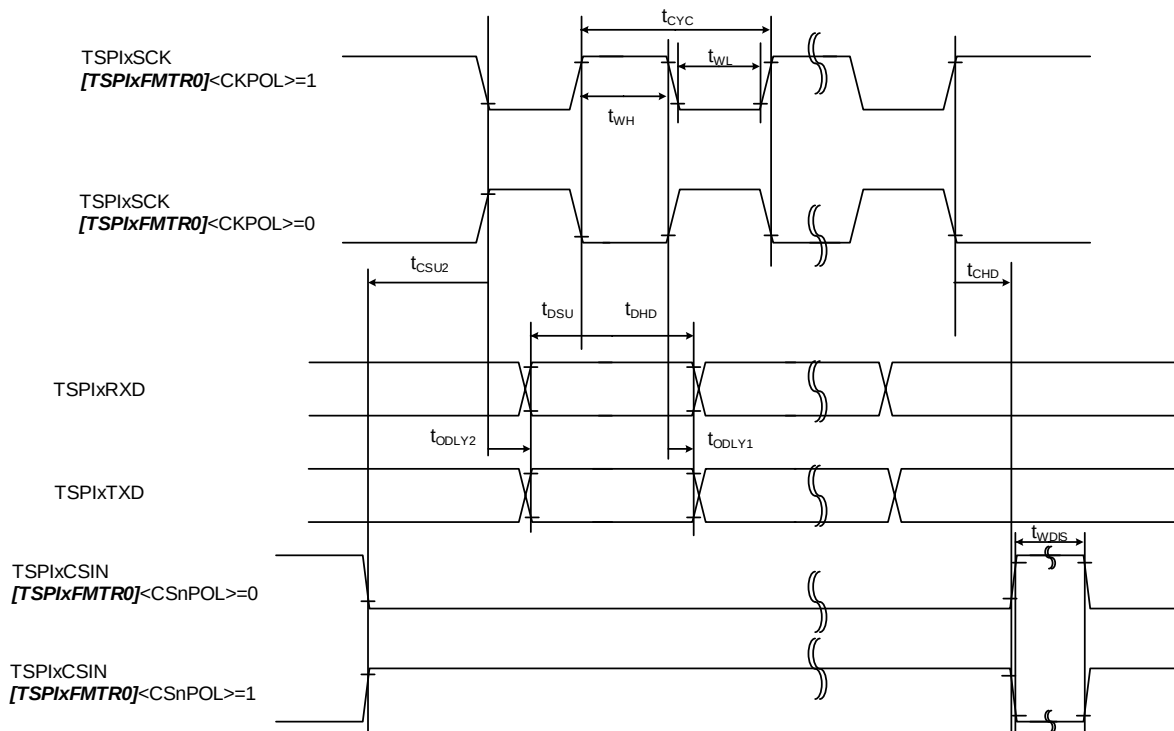
図 7.6 2ndクロックエッジサンプリング(スレーブ)
