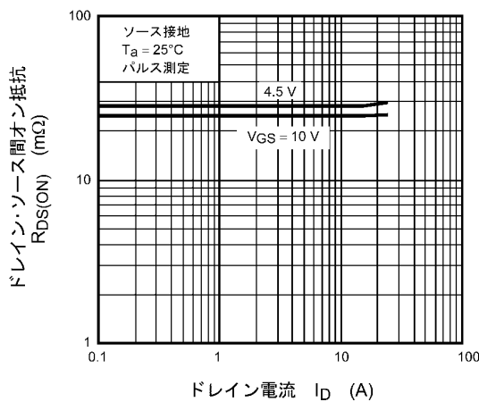
図 8.2.5 R_{DS(ON)} - I_D
