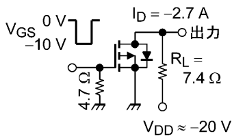
図 6.2.1 スwitchング時間の測定回路例 (P-ch) 図 6.2.2 スwitchング時間の測定回路例 (N-ch)
