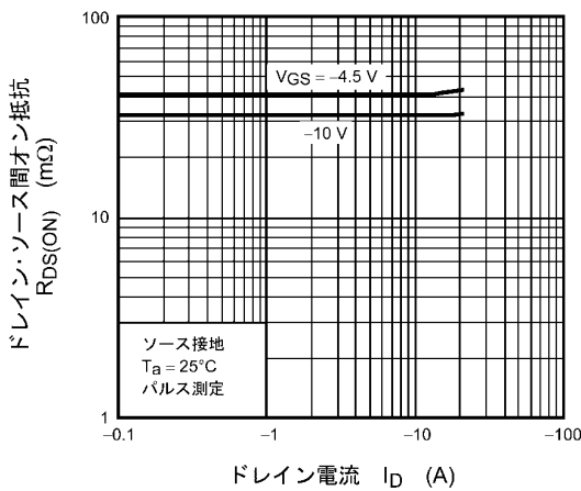
図 8.1.5 R_{DS(ON)} - I_D
