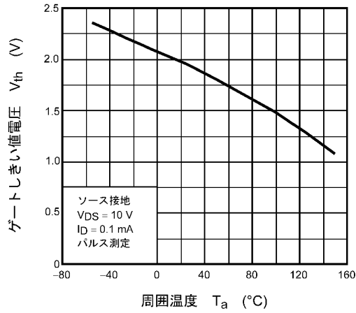
図 8.2.9 V_{th} - T_a
