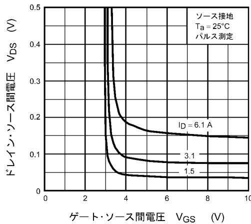
図 8.2.4 V_{DS} - V_{GS}
