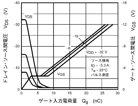
図 8.1.10 ダイナミック入出力特性
