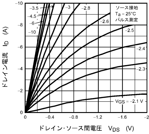
図 8.1.1 I_D - V_{DS}
