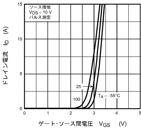
図 8.2.3 I_D - V_{GS}
