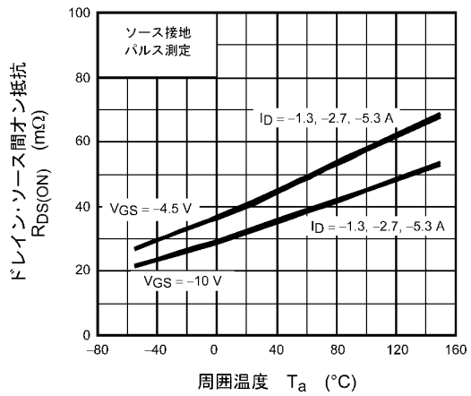
図 8.1.6 R_{DS(ON)} - T_a
