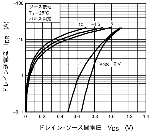
図 8.1.7 I_{DR} - V_{DS}
