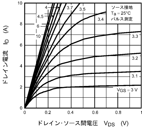
図 8.2.1 I_D - V_{DS}
