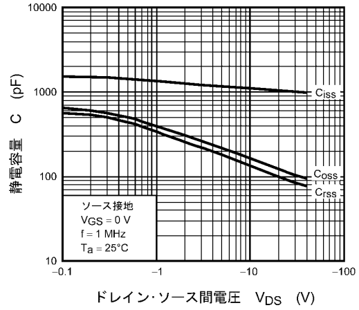
図 8.1.8 静電容量 - V_{DS}
