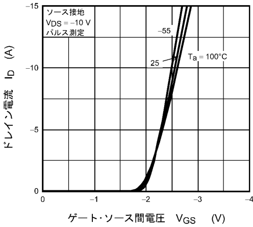
図 8.1.3 I_D - V_{GS}
