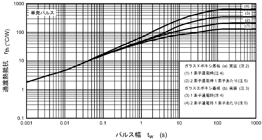
図 8.1.12 r_{th} - t_w (最大値 (保証値))
