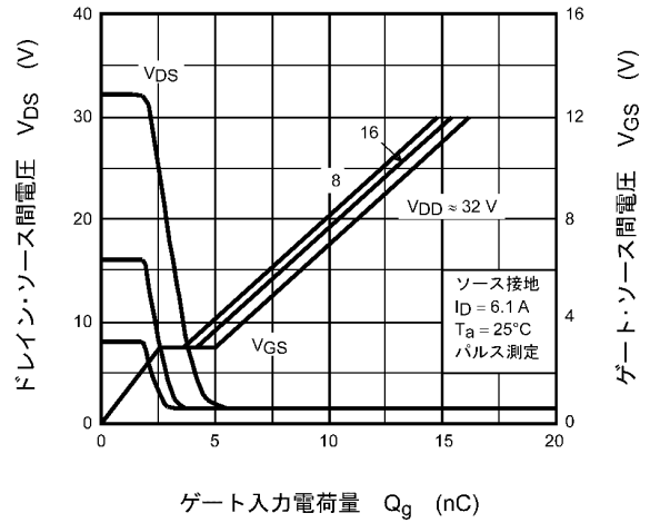
図 8.2.10 ダイナミック入出力特性
