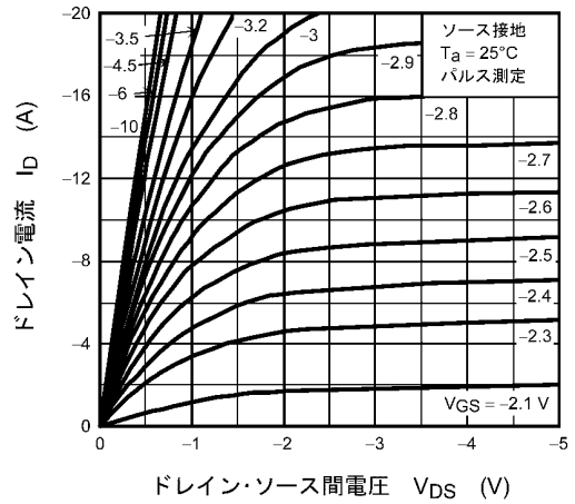
図 8.1.2 I_D - V_{DS}
