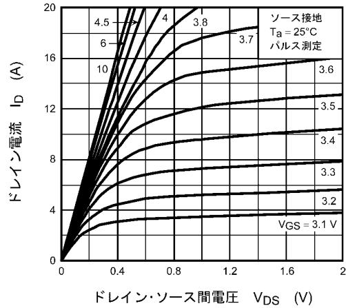
図 8.2.2 I_D - V_{DS}
