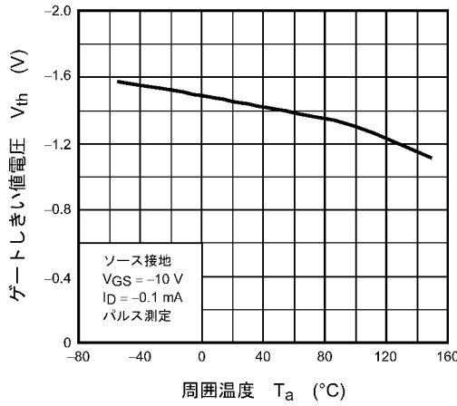
図 8.1.9 V_{th} - T_a
