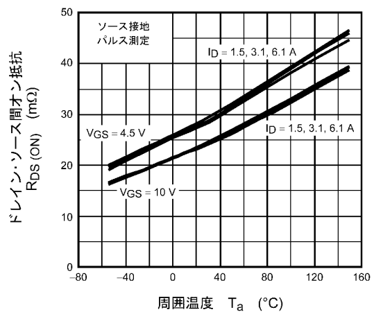
図 8.2.6 R_{DS(ON)} - T_a
