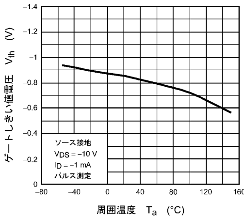
図 8.9 V_{th} - T_a
