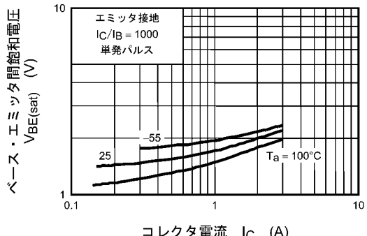
図 8.1.5 VBE(sat) - IC
