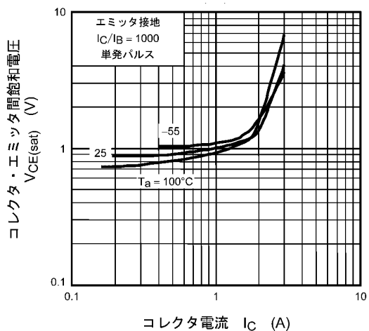
図 8.1.3 VCE(sat) - IC
