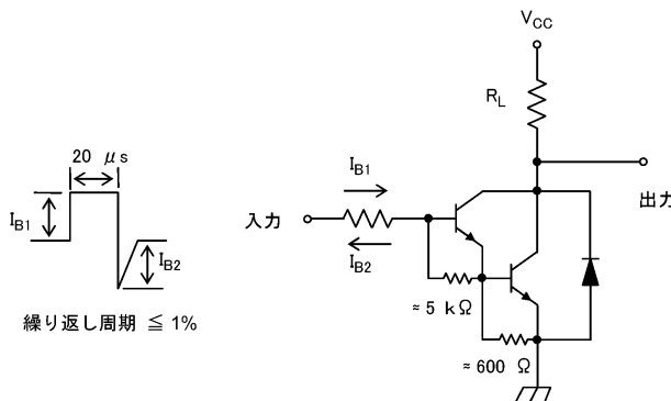
図 5.1.1 スwitching時間測定回路
