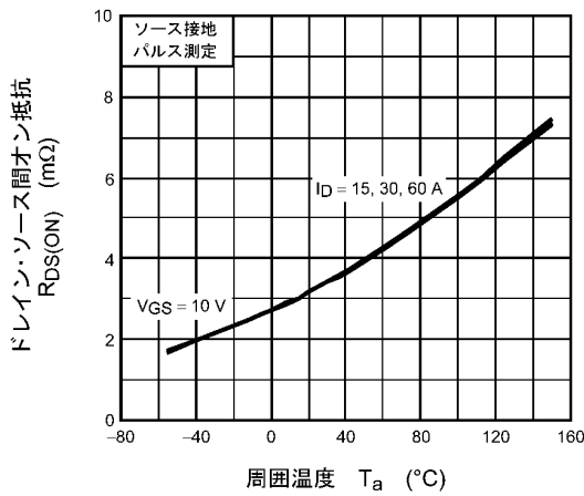
図 8.9 R_{DS(ON)} - T_a
