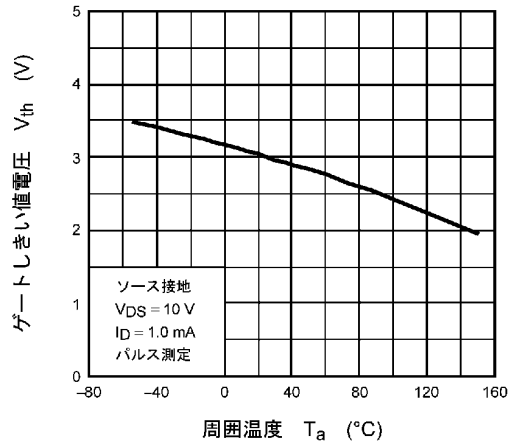
図 8.8 V_{th} - T_a
