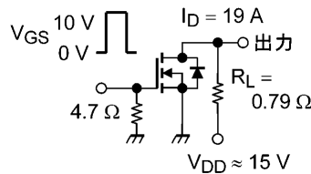
図 6.2.1 スwitchング時間の測定回路例
