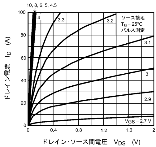
図 8.2 I_D - V_{DS}
