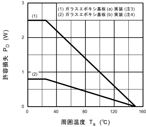
周囲温度 T_a (°C) 図 8.14 P_D - T_a (最大値 (保証値))
