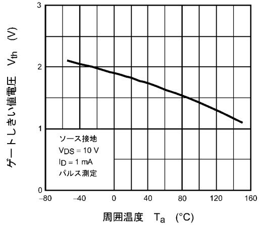
図 8.8 V_{th} - T_a
