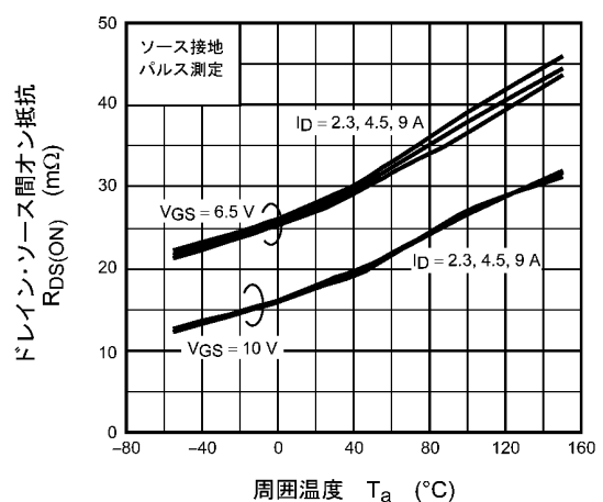
図 8.6 R_{DS(ON)} - T_a
