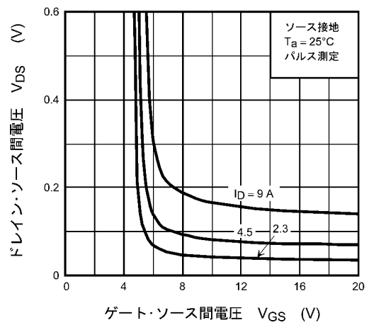
図 8.4 V_{DS} - V_{GS}
