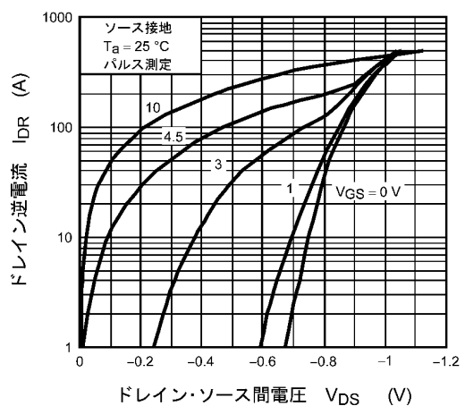
図 8.6 I_{DR} - V_{DS}
