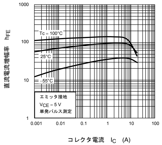
h_{FE} - I_C
