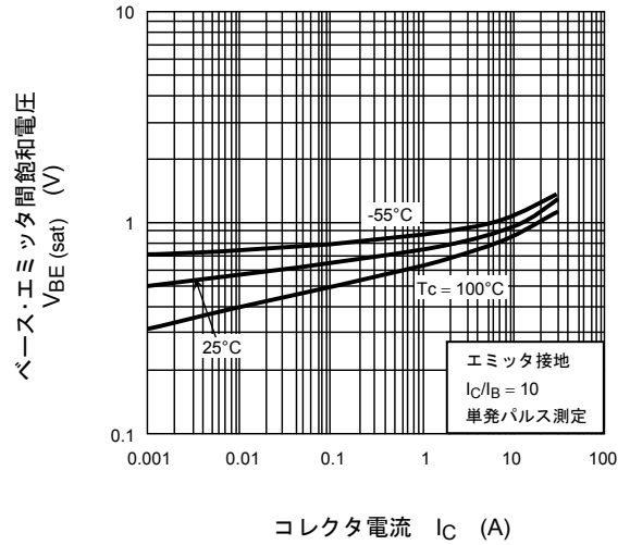
V_{BE(sat)} - I_C
