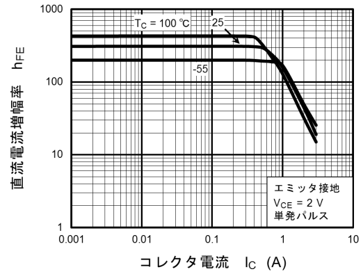
図 7.2 h_{FE} - I_c
