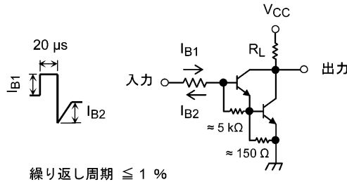
図 5.2.1 スwitching時間の測定回路
