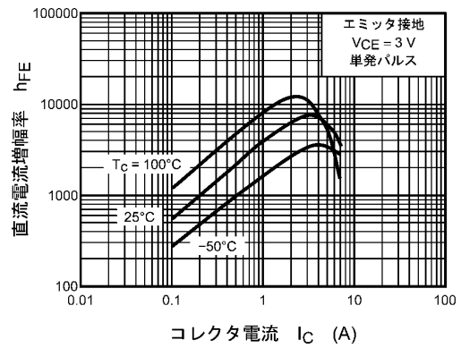
図 7.4 h_{FE} - I_C
