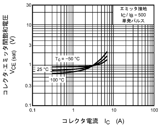
図 7.5 V_{CE(sat)} - I_C
