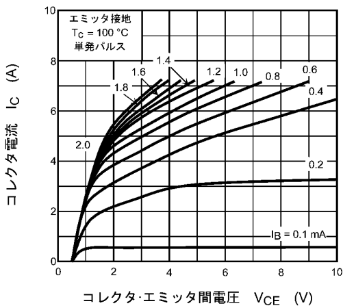
図 7.3 I_C - V_{CE}
