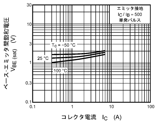
図 7.6 V_{BE(sat)} - I_C
