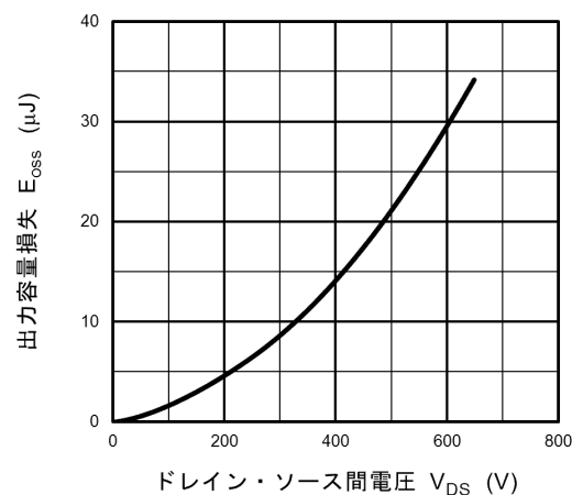
図 8.14 E_{oss} - V_{DS}
