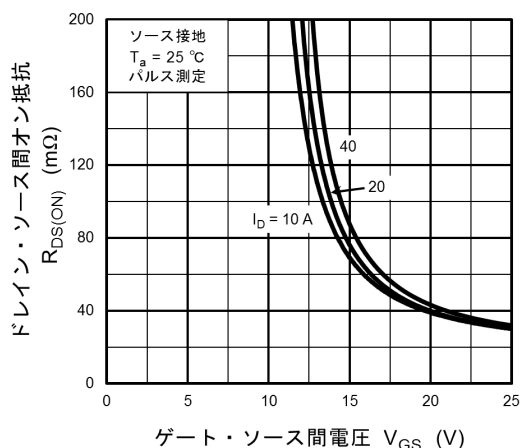
図 8.8 R_{DS(ON)} - V_{GS}
