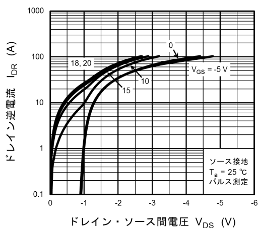
図 8.9 I_{DR} - V_{DS}
