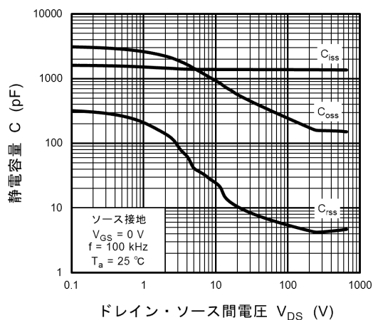
図 8.13 C - V_{DS}
