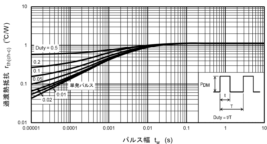
図 8.15 r_{th(ch-c)} - t_w (最大値 (保証値))
