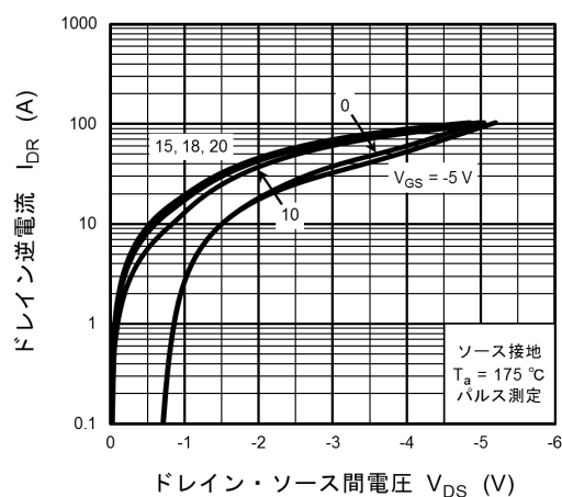
図 8.10 I_{DR} - V_{DS}
