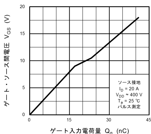
図 8.12 ダイナミック入力特性
