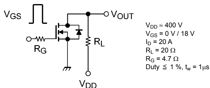
図 6.2.1 スwitchング時間の測定回路
