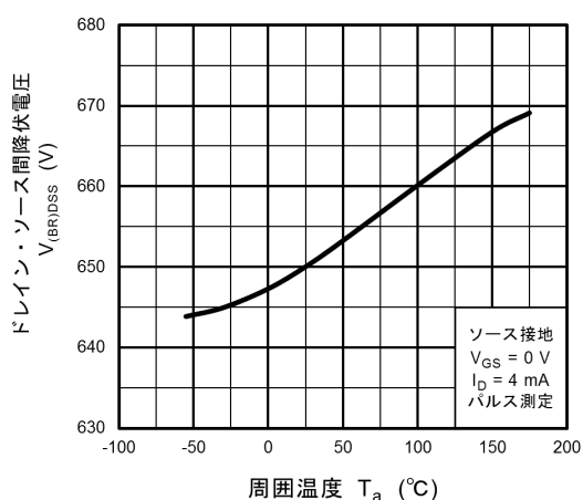
図 8.11 V_{DS(ON)} - T_a
