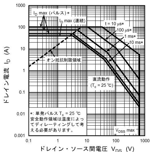
図 8.16 安全動作領域 (最大値 (保証値))
