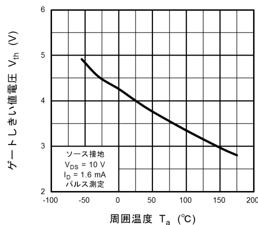
図 8.4 V_{th} - T_a
