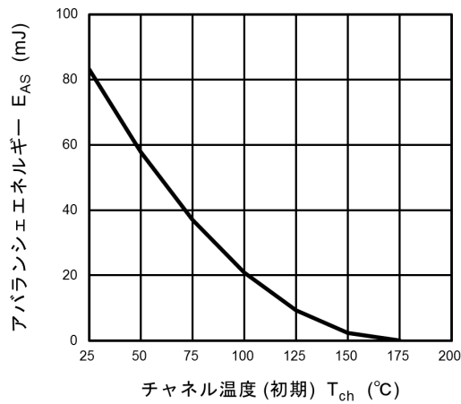
図 8.15 E_{AS} - T_{ch}
